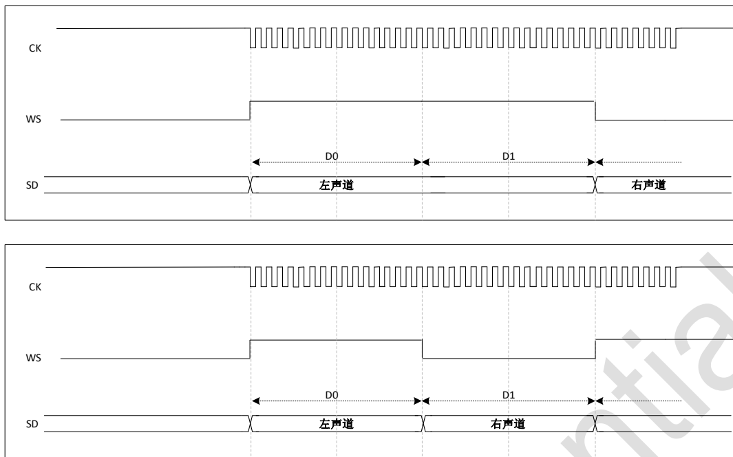
图 34-19 I²S MSB 对齐标准 (16/32 全精度, CKPOL=1)
