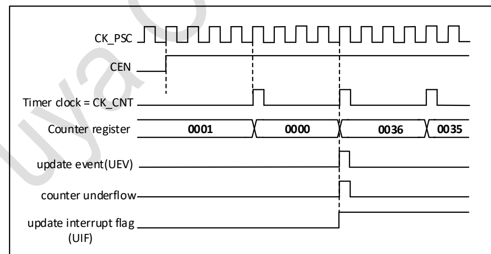
图 18-12 计数器时序图，内部时钟 4 分频
