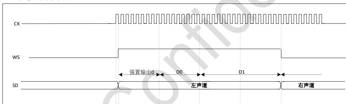
图 34-26 I²S LSB 对齐标准(24 位帧, CKPOL=0)
