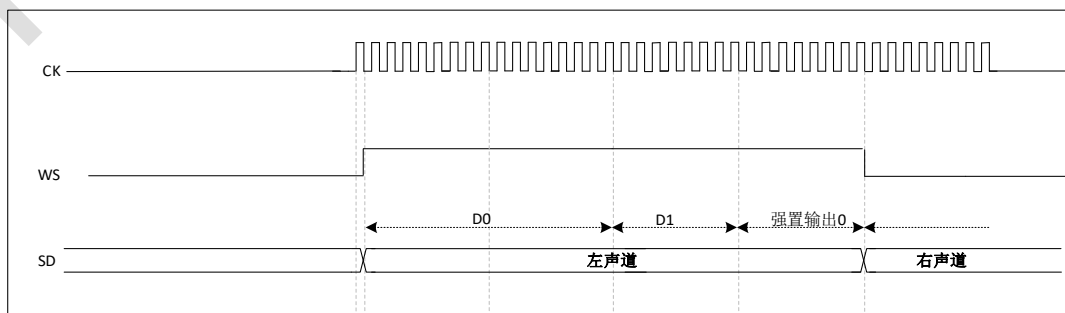
图 34-22 I²S MSB 对齐标准(16 位扩展到 32 位, CKPOL=0)
