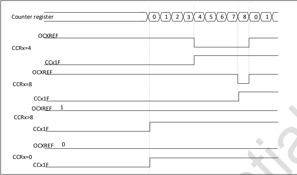
图 18-34 边沿对齐方式 PWM 输出波形 (ARR=8)
