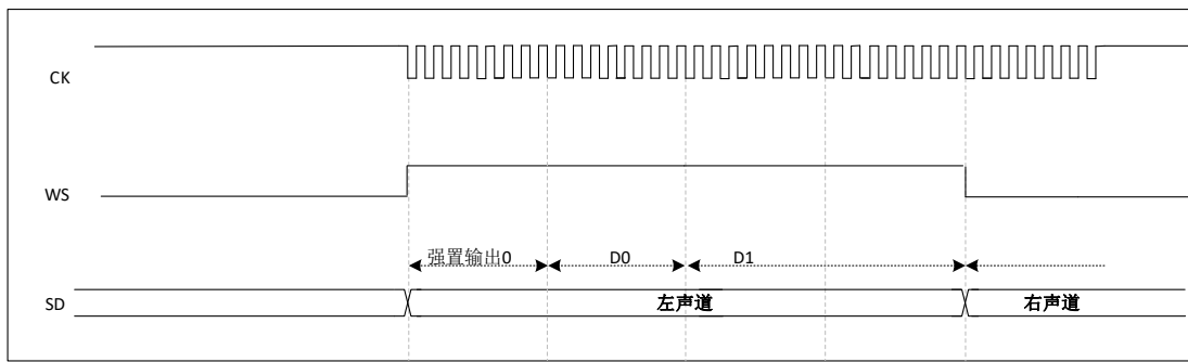
图 34-23 I²S MSB 对齐标准(16 位扩展到 32 位, CKPOL=1)
