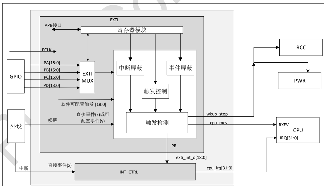
图 11-1 EXTI 框图
