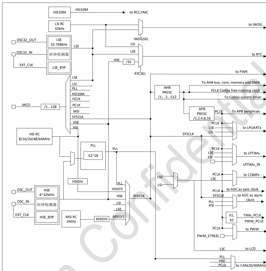
图 6-2 时钟结构
