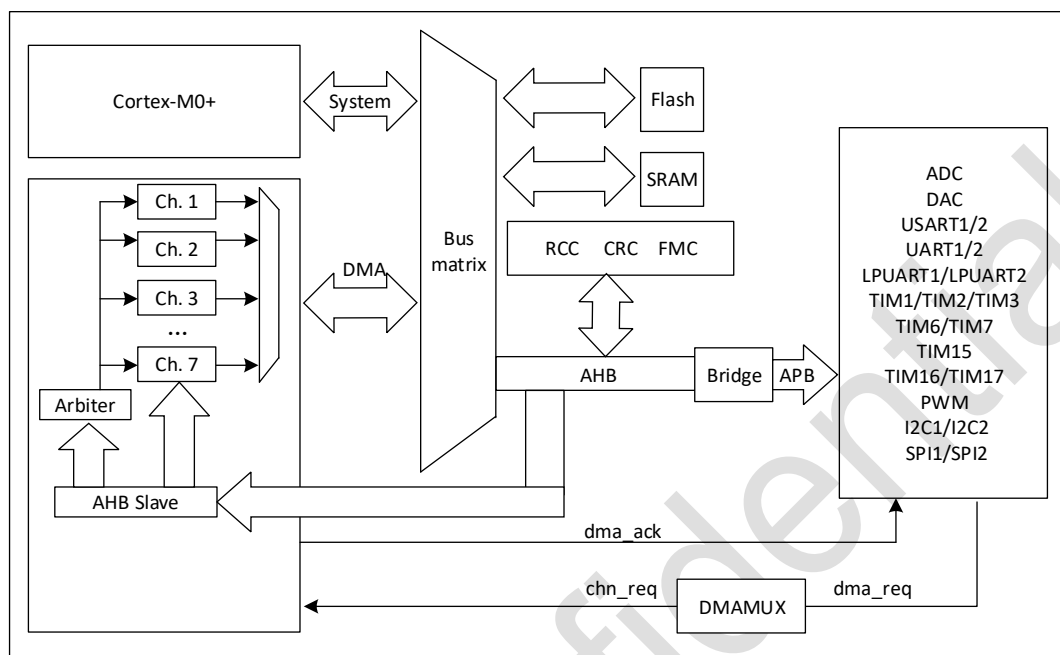
图 10-1 DMA 框图
