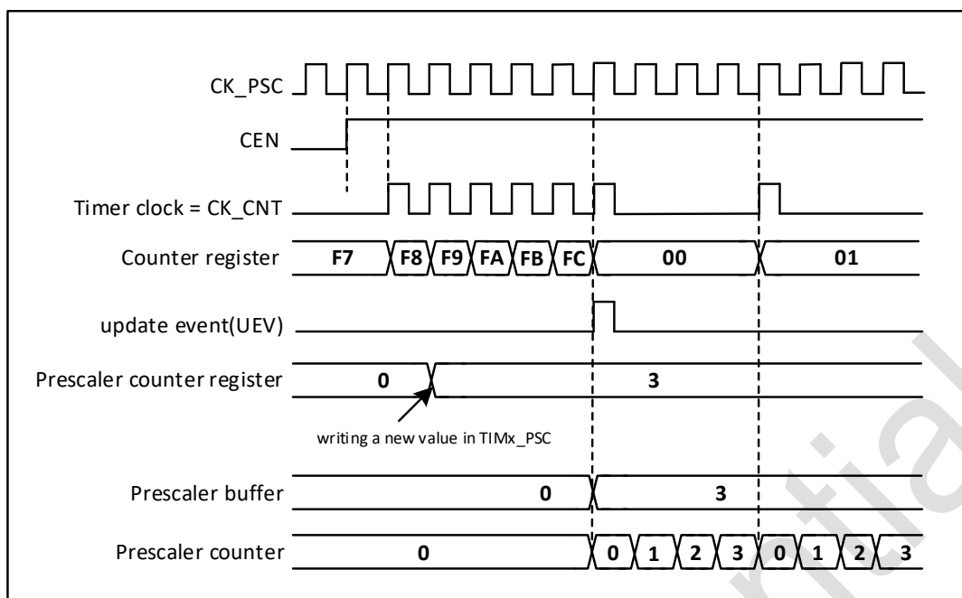
图 21-3 预分频器分频由 1 变为 4 时的计数器时序图
