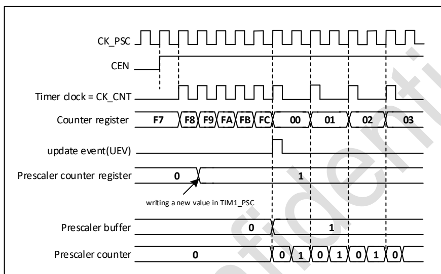
图 18-2 预分频器分频由 1 变为 2 时的计数器时序图
