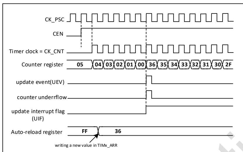
图 19-14 计数器时序图，未使用重复计数器时更新事件
