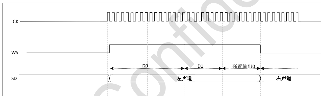
图 34-20 I²S MSB 对齐标准(24 位帧, CKPOL=0)
