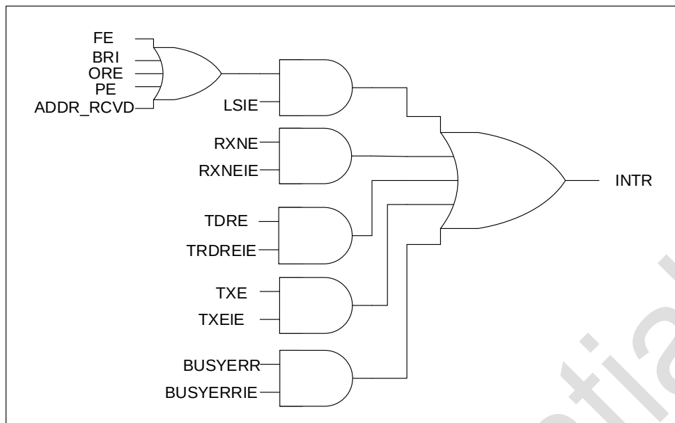
图 32-8 中断映射图
