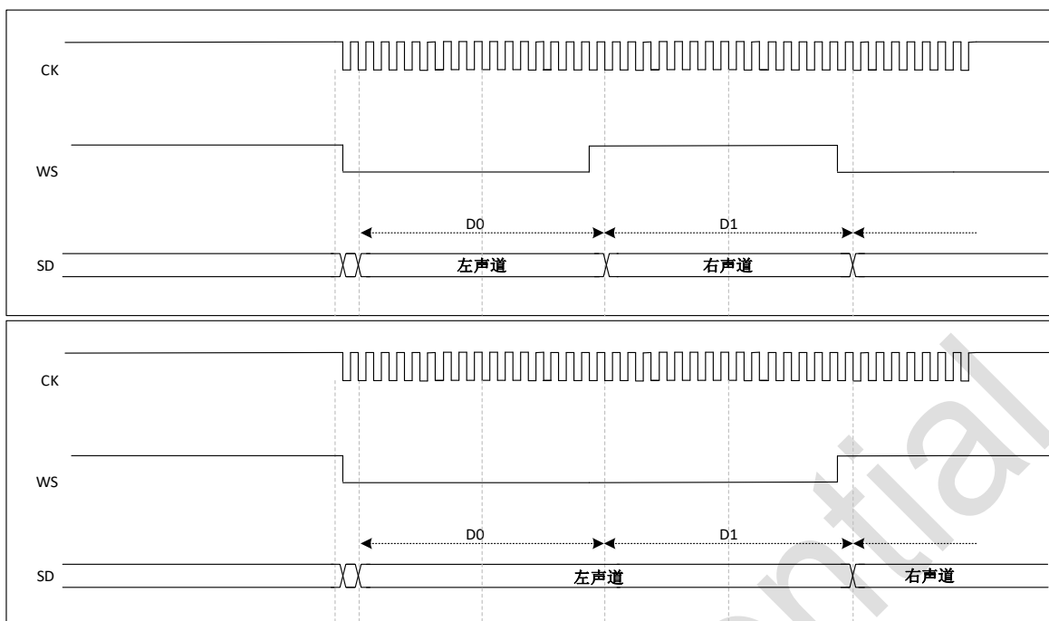
图 34-14 I²S 飞利浦协议波形 (16/32 位全精度, CKPOL=1)
