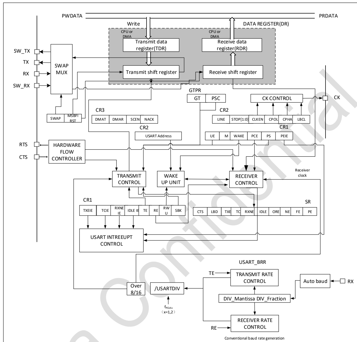
图 31-1 USART 框图
