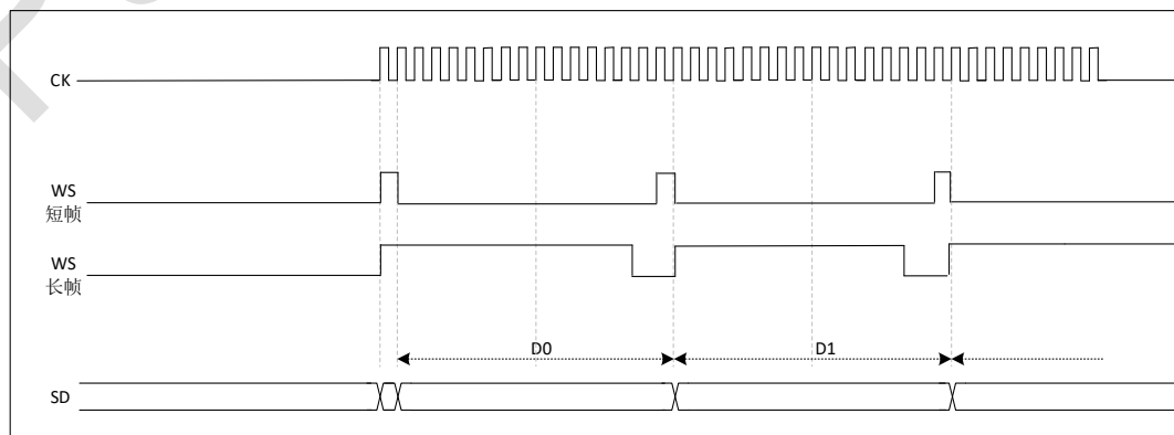
图 34-30 I²S PCM 标准(16 位帧, CKPOL=0)
