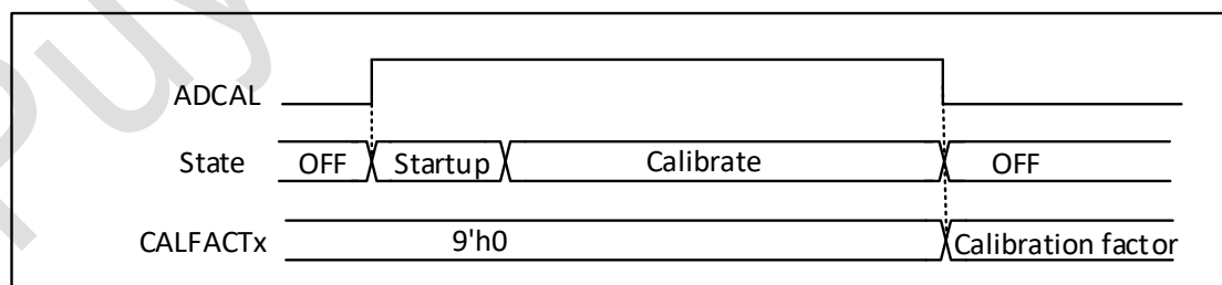
图 13-3 ADC 校准
