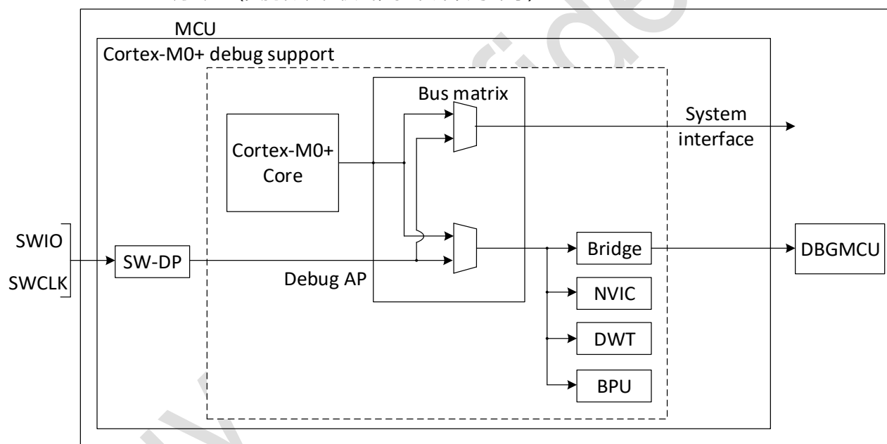
图 37-1 DBG 框图
