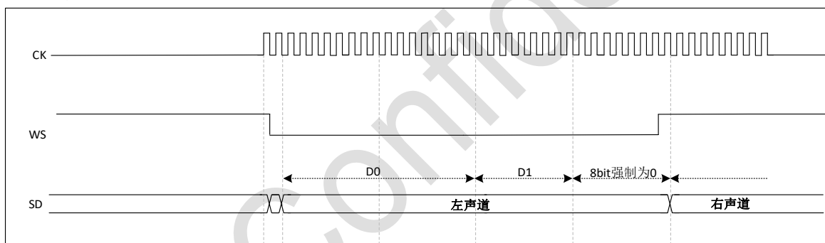
图 34-15 I²S 飞利浦协议波形(24 位帧, CKPOL=0)
