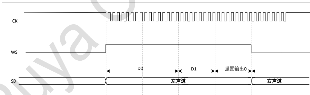
图 34-21 I²S MSB 对齐标准(24 位帧, CKPOL=1)
