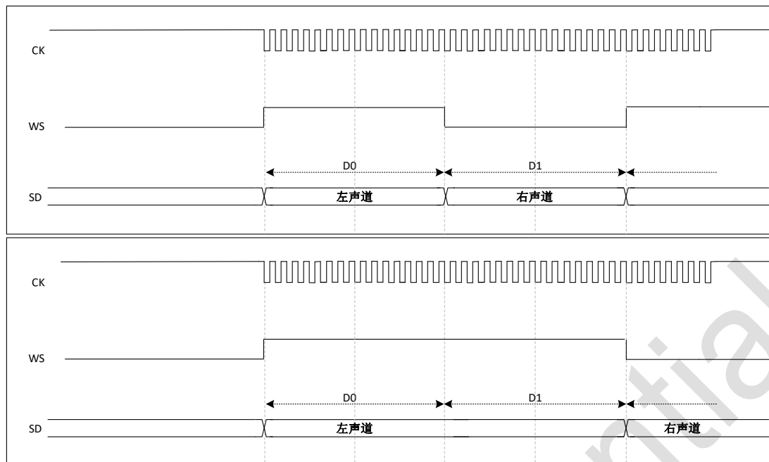
图 34-25 I²S LSB 对齐标准 (16/32 位全精度, CKPOL=1)
