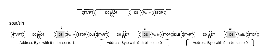
图 32-5 9位字符
