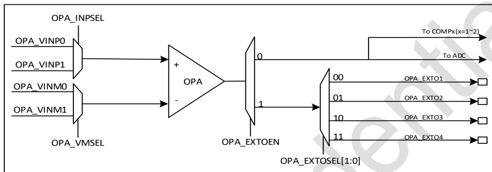
图 16-1 OPA 框图
