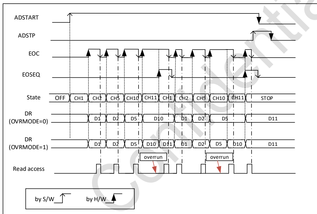
图 13-18 过载
