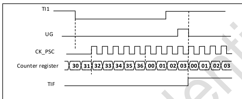
图 20-28 复位模式下的控制电路
