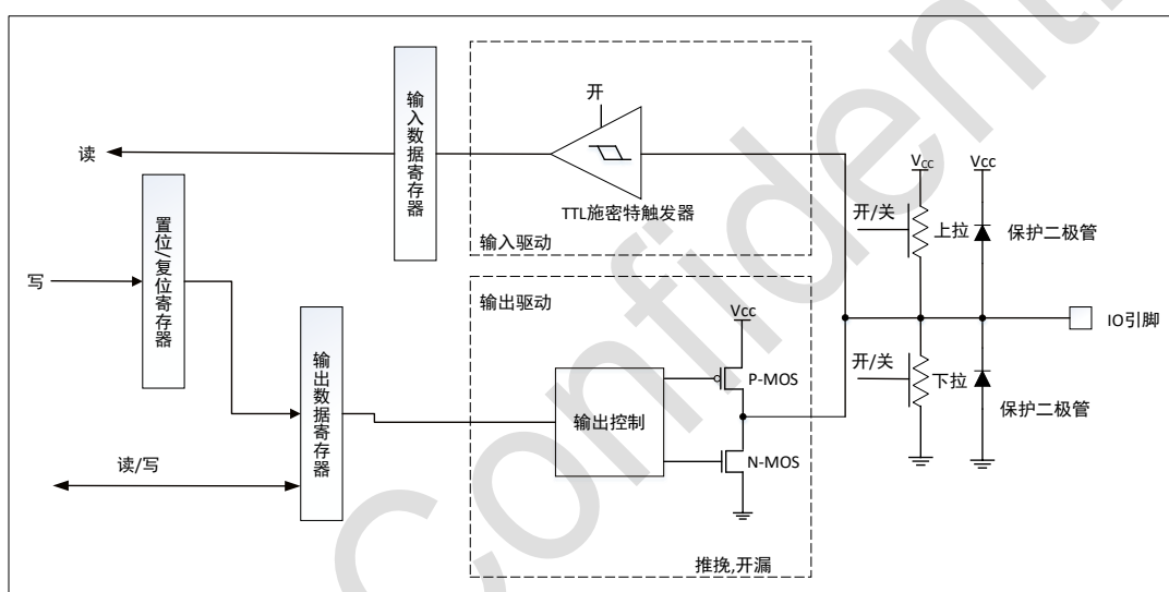
图 7-3 输出配置
