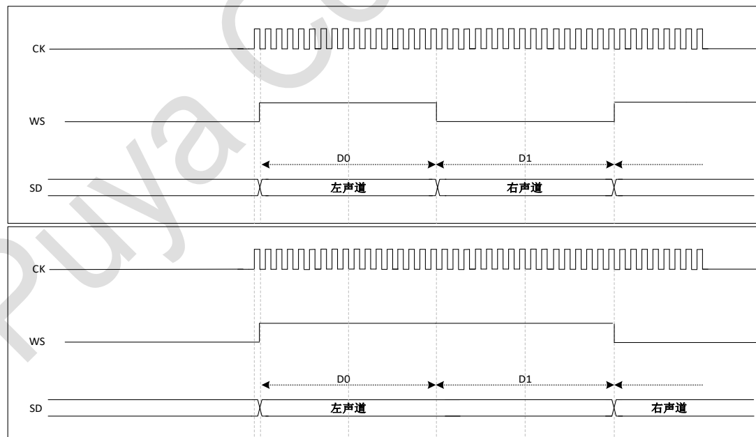
图 34-18 I²S MSB 对齐标准 (16/32 全精度, CKPOL=0)
