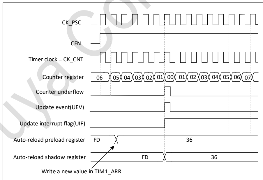
图 18-19 计数器时序图，ARPE=1 时的更新事件(计数器下溢)
