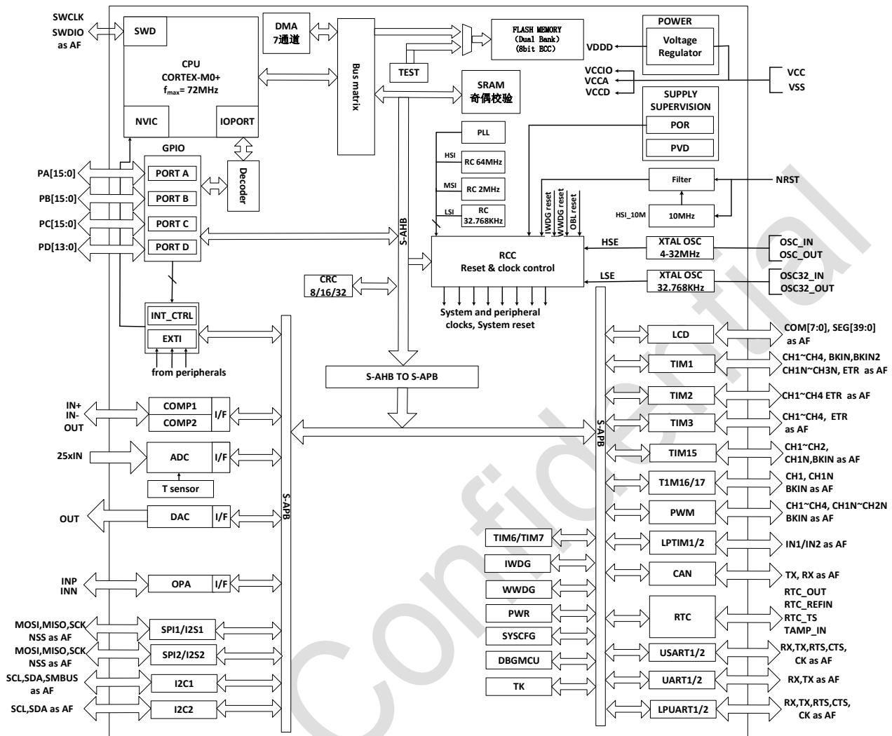
图 2-1 系统框图
