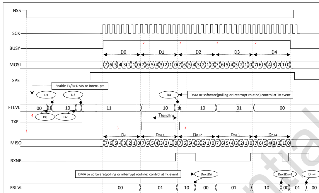
图 34-9 主模式全双工通讯(帧长=8)
