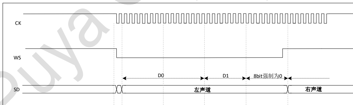
图 34-16 I²S 飞利浦协议波形(24 位帧, CKPOL=1)
