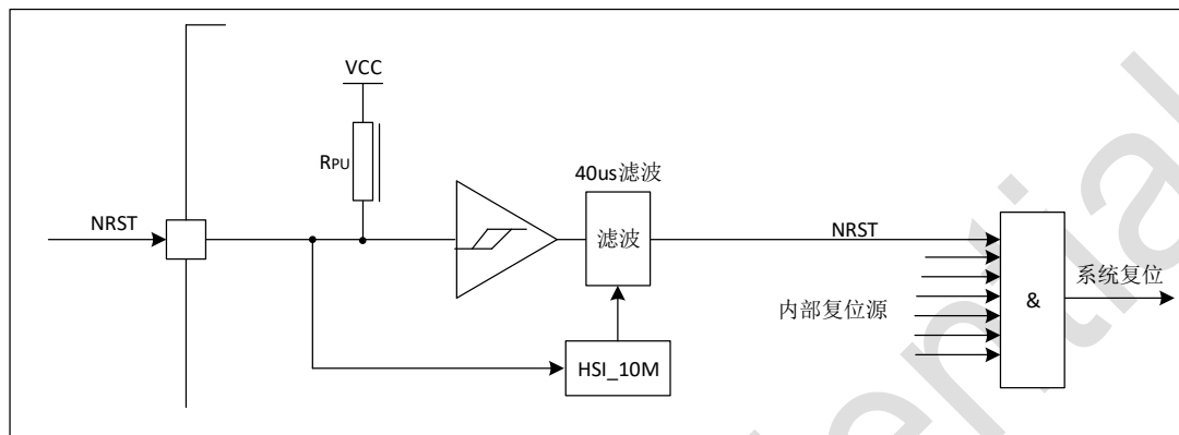
图 6-1 复位电路
