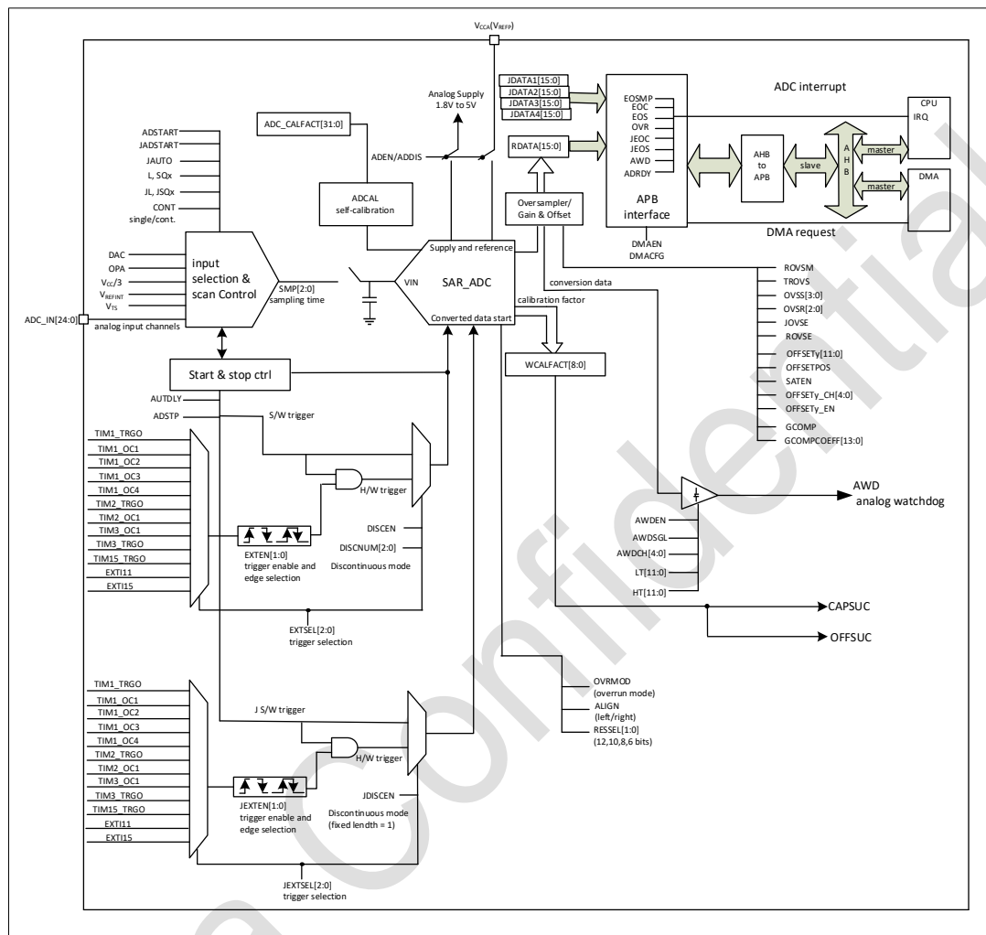
图 13-1 ADC 框图
