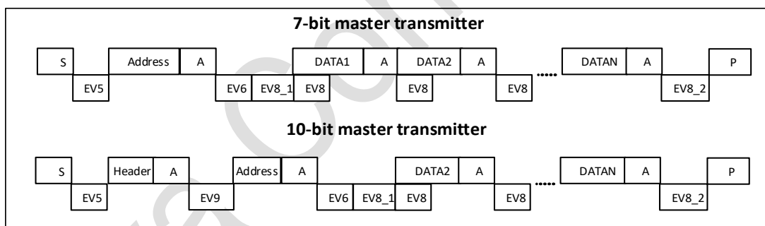
图 30-5 主机发送序列图
