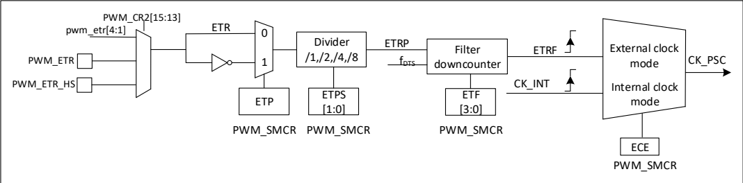
图 23-17 外部触发输入框图
