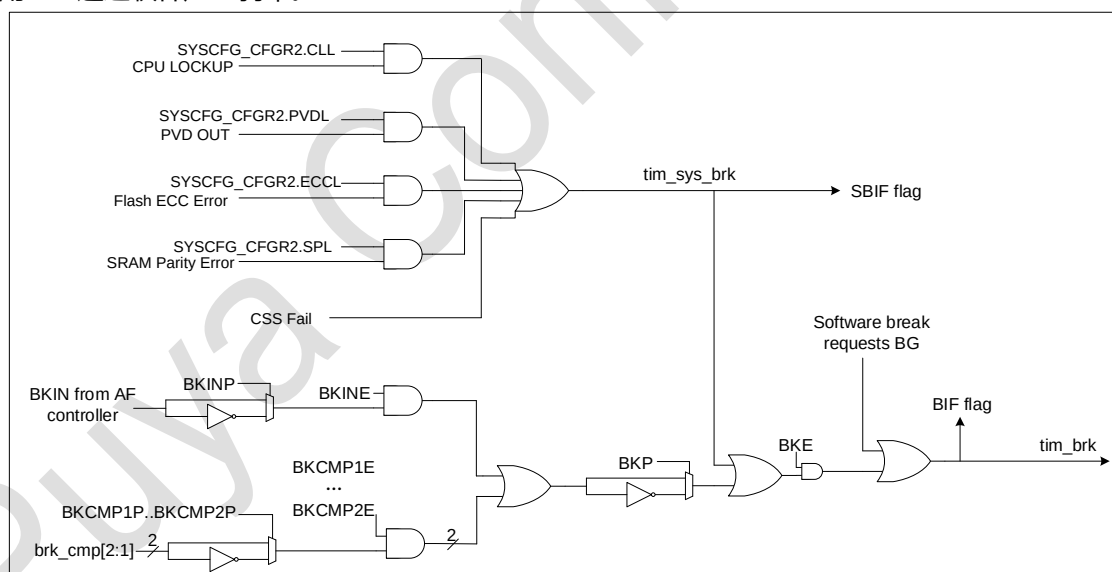
图 18-39 刹车电路图
