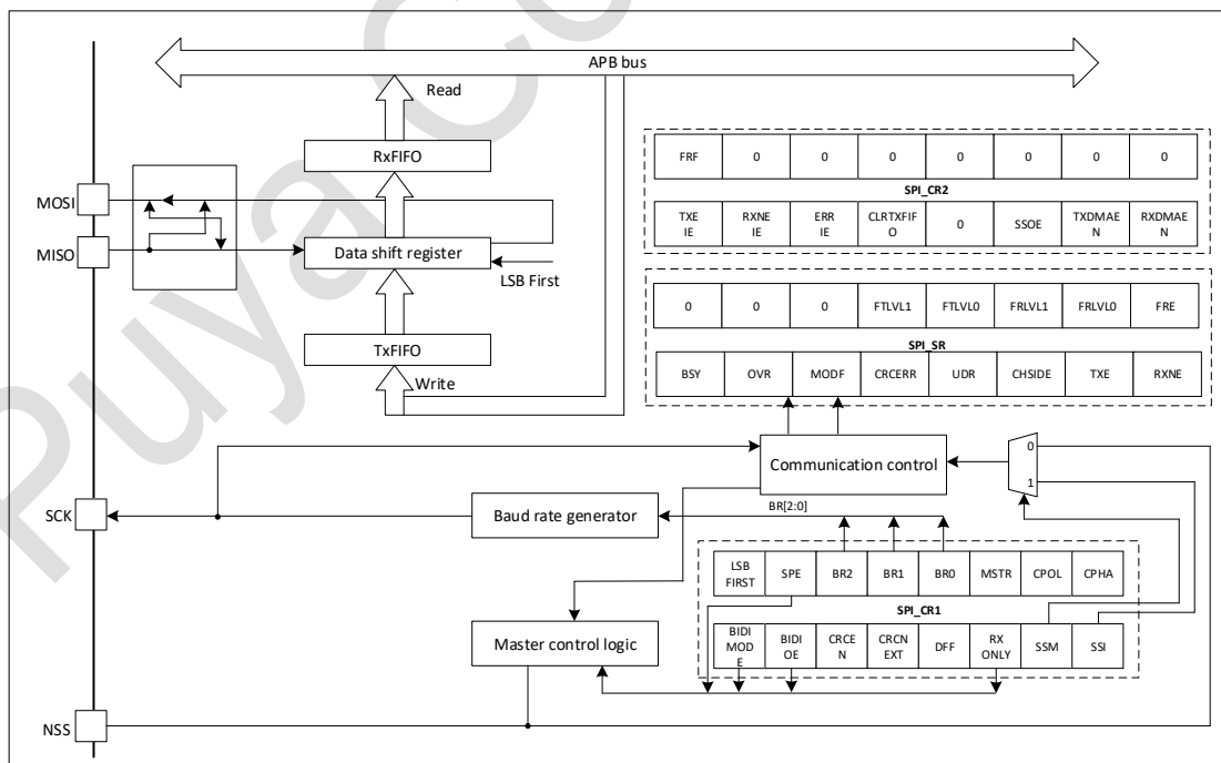
图 34-1 SPI 框图
