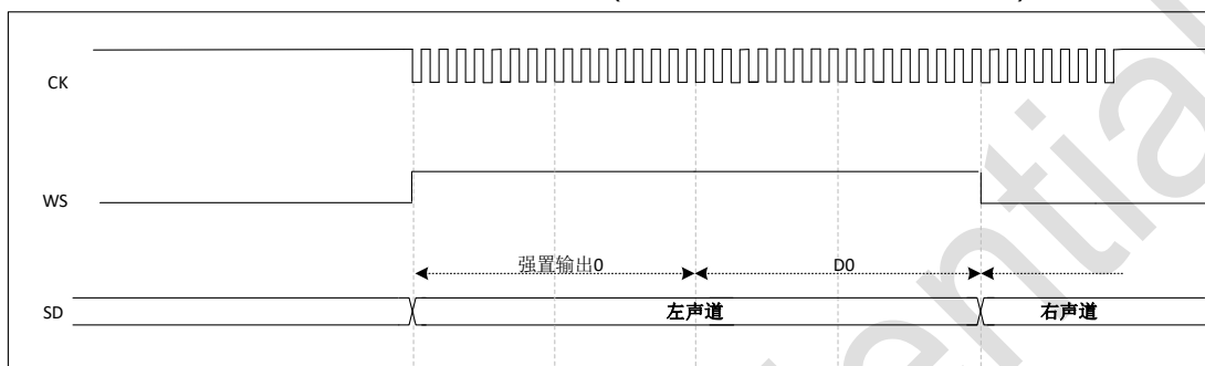
图 34-29 I²S LSB 对齐标准(16 位扩展到 32 位, CKPOL=1)
