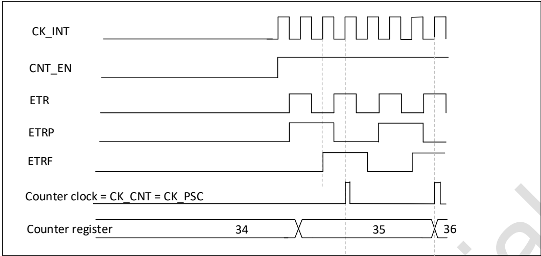
图 18-27 外部时钟模式 2 控制电路时序
