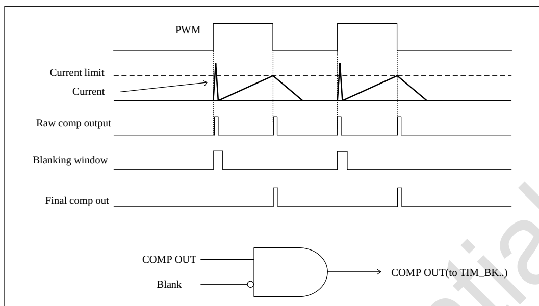
图 15-3 COMP 消隐
