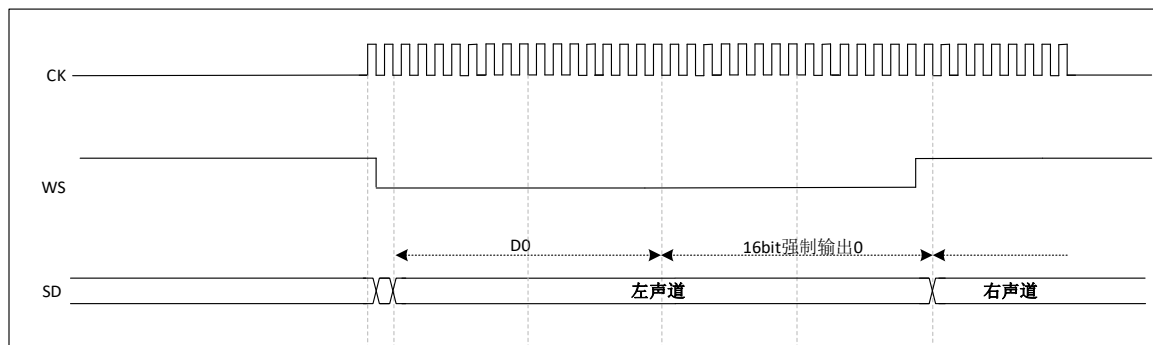
图 34-17 I²S 飞利浦协议波形(16 位扩展到 32 位)
