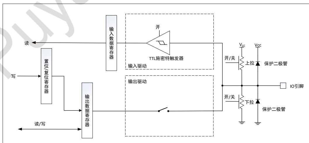
图 7-2 输入浮空/上拉/下拉配置
