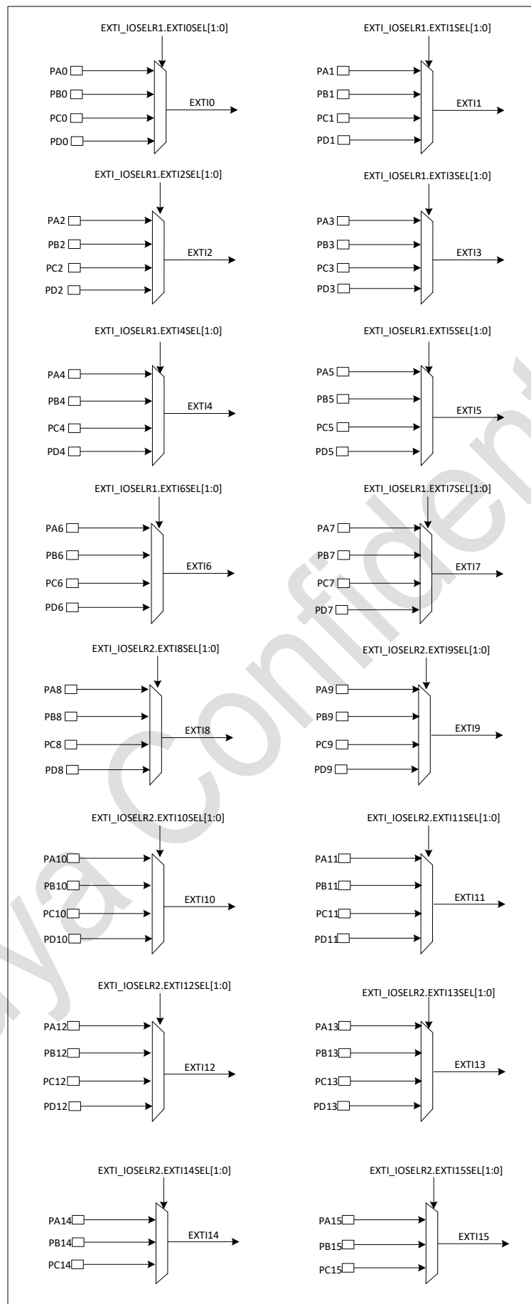
图 11-2 EXTI GPIO 复用
