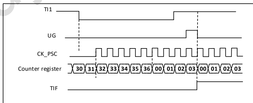
图 19-37 复位模式下的控制电路
