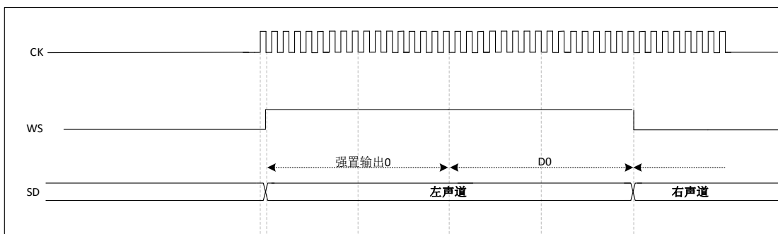
图 34-28 I²S LSB 对齐标准(16 位扩展到 32 位, CKPOL=0)
