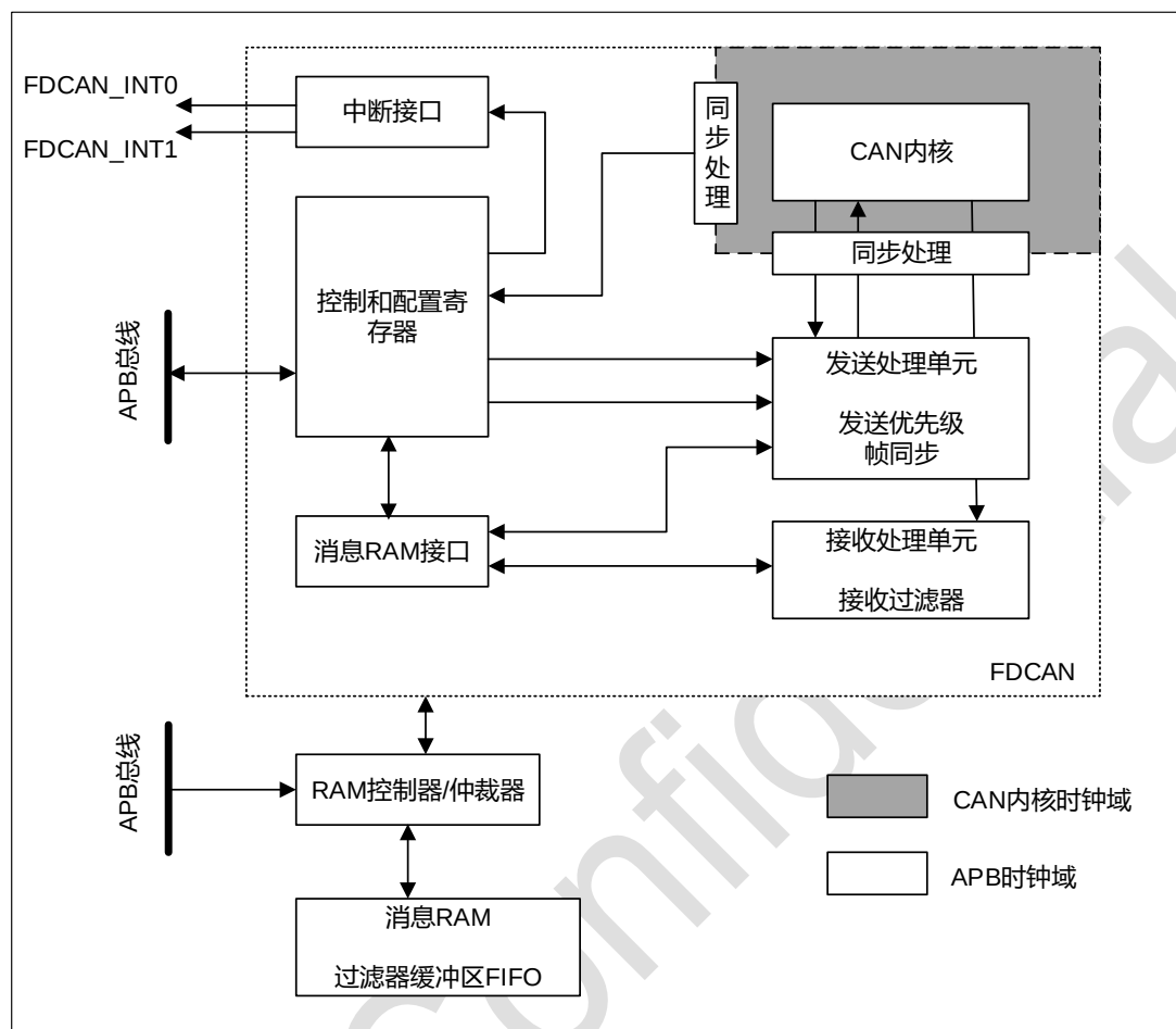
图 36-1 FDCAN 框图
