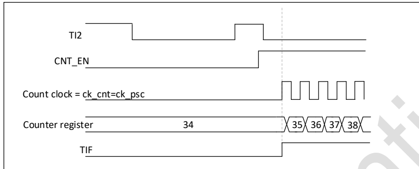
图 18-50 触发模式下的控制电路
