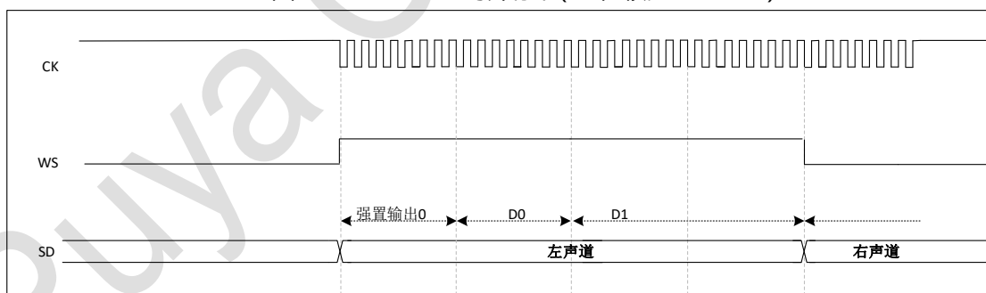
图 34-27 I²S LSB 对齐标准(24 位帧, CKPOL=1)
